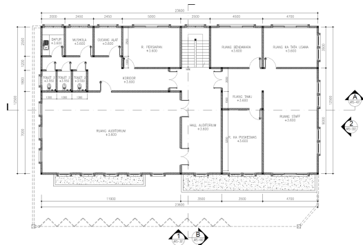
Gambar 1. Denah Rencana
