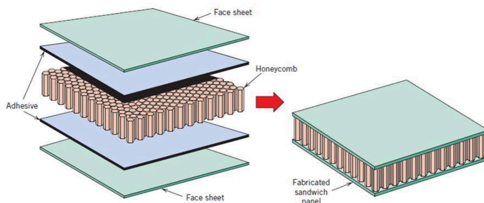
GAMBAR 1. KOMPOSIT HYBRID
