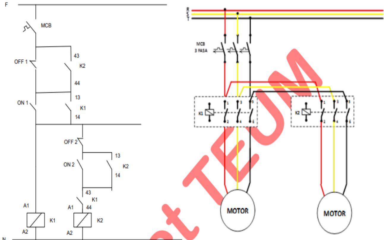
Gambar rangkaian kendali dan rangkaian utama 2 motor yang bekerja secara berurutan
