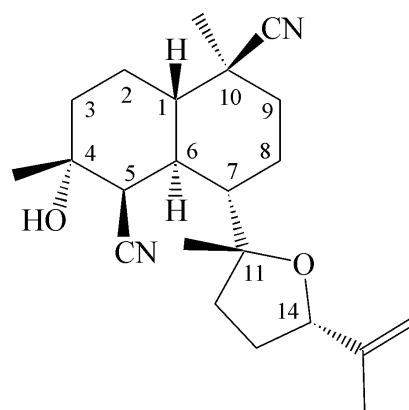
Kalihinol C
