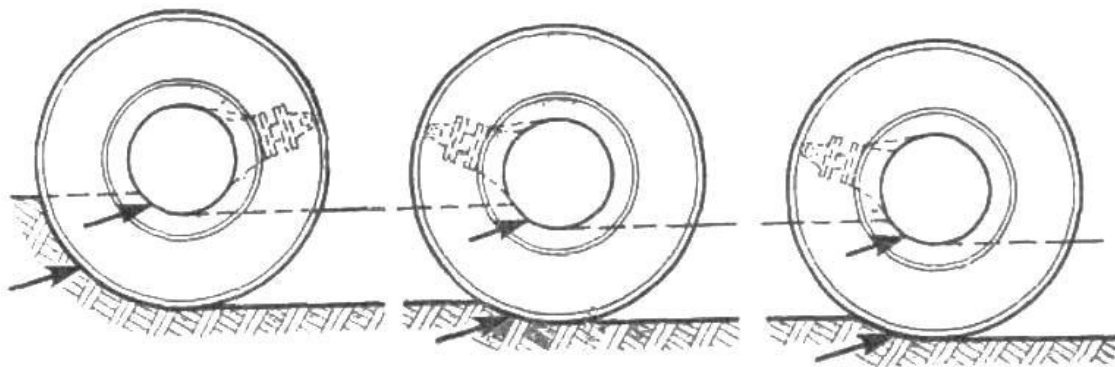
Рис. 11. Упрощенная схема сил, оказывающих сопротивление движению колес трехосного автомобиля на глубоком снегу
