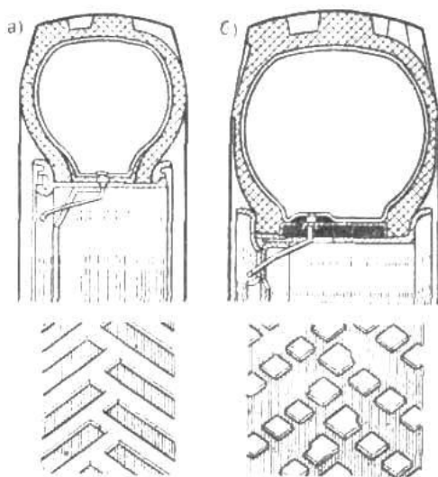
Рис. 6. Сечение шины и ее рисунок протектора:
