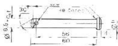
Рис. 18. Предохранительный палец лебедки
