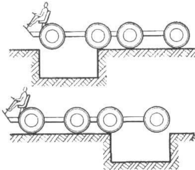
Рис. 25. Схема преодоления рва четырехосным автомобилем.
