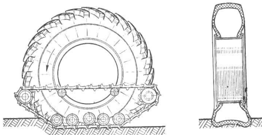
Рис. 7. Характер взаимодействия деформированной шины с грунтом 20
