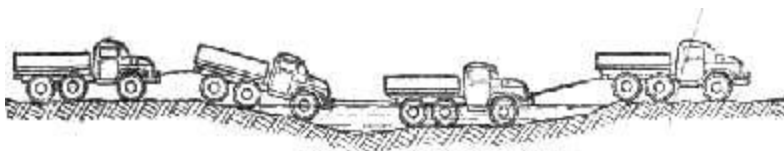
Рис. 15. Преодоление брода несколькими автомобилями, сцепленными между собой
