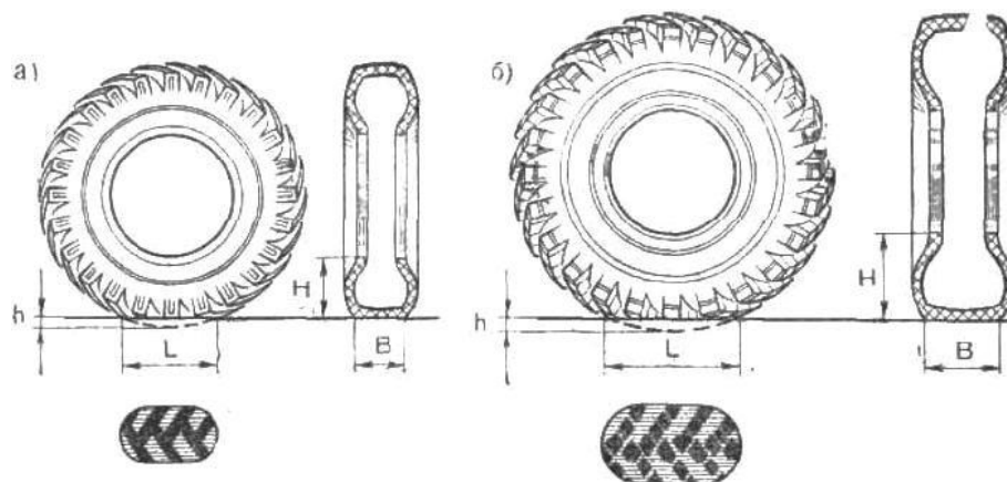
Рис. 4. Шина: а — обычная; б — увеличенного профиля
