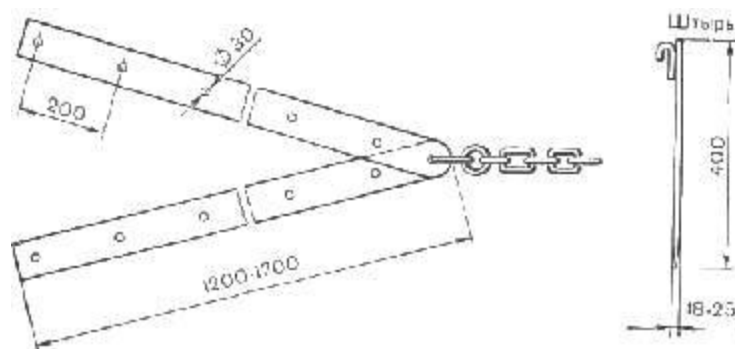
Рис. 20. Якорное устройство
