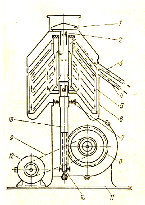
Рис.6. Структурно-кінематична схема сепаратора СОМ-3-1000:
