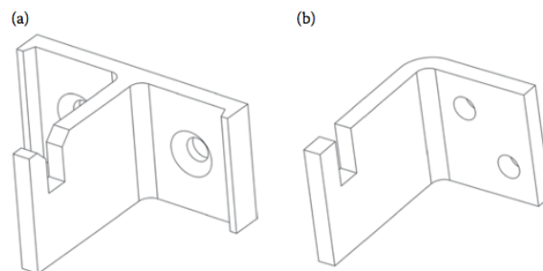
Gambar SEQ Gambar \* ARABIC 1. Desain Bracket (Sumber: Jamnia, 2018)
