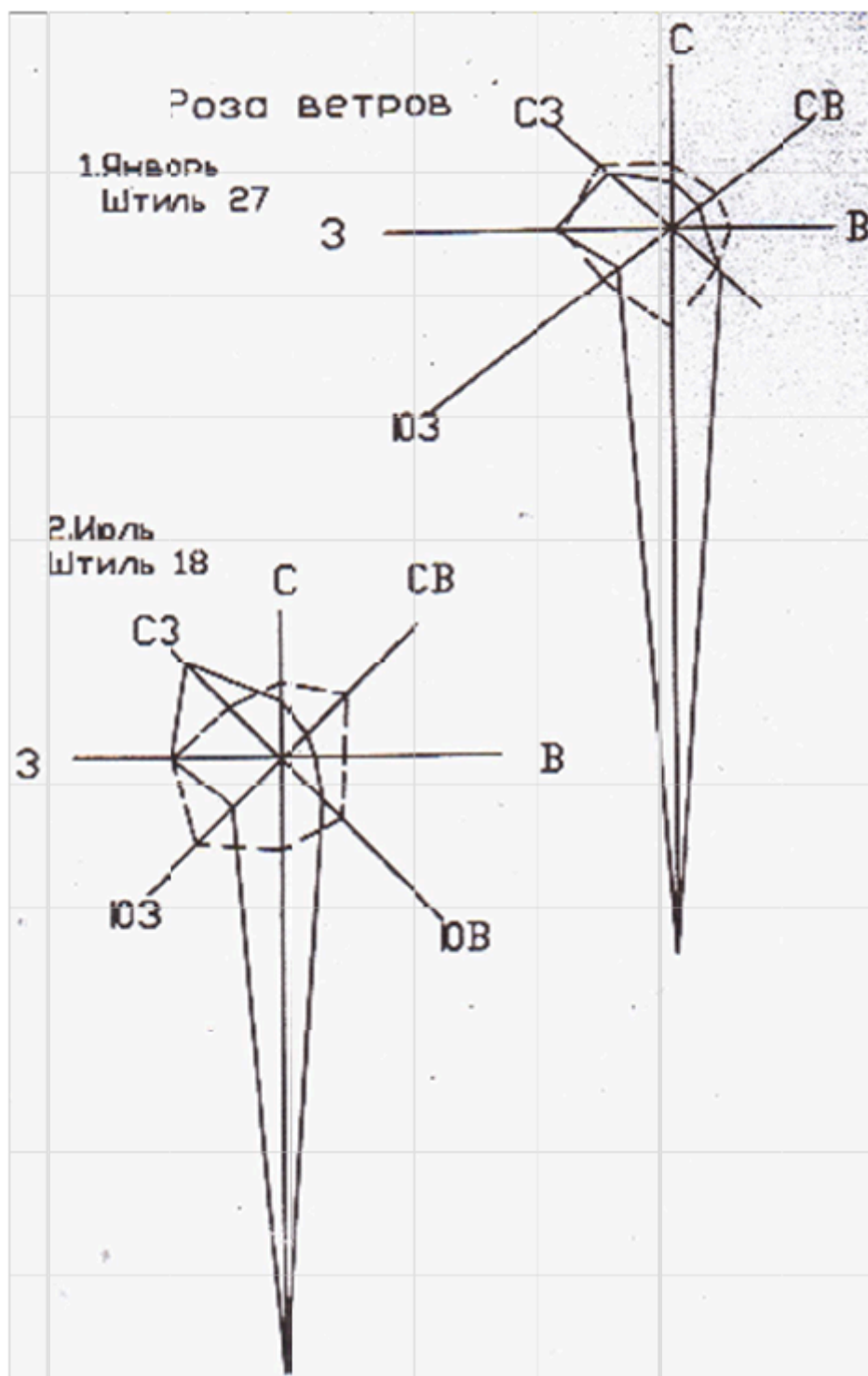
Рис. 3. Роза ветров в г. Кызыл-Кия
