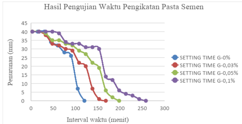
Gambar 3 Pengaruh persentase penambahan gula terhadap waktu ikat pasta semen [Times New Roman, 11]
