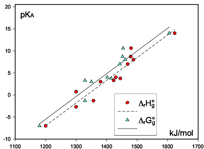
Figure 1 : pK_A en solution aqueuse en fonction de \Delta_r H_g^\circ et \Delta_r G_g^\circ de quelques oxoacides.
