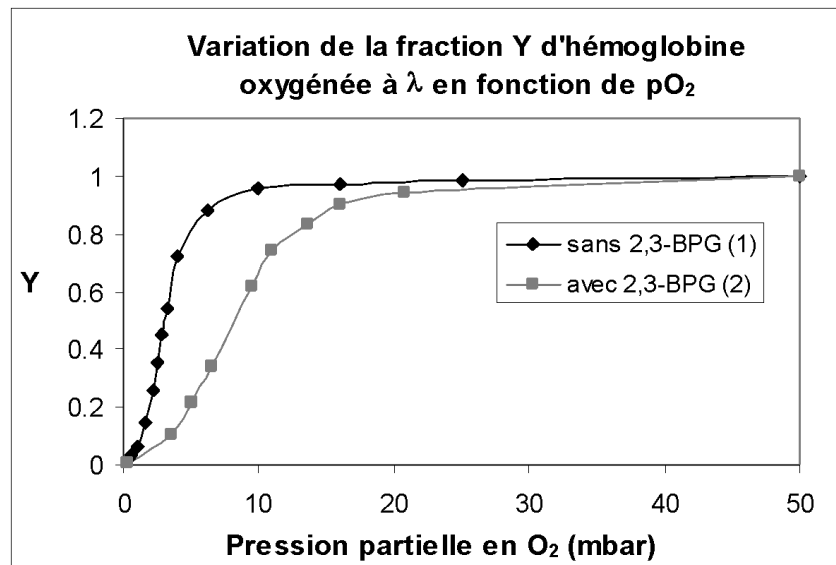
Graphe 4 : Variation de Y pour des solutions 1 et 2 en fonction de pO_2 .
