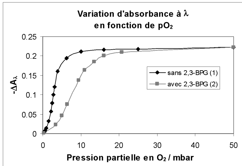
Graph 3 : Variation d'absorbance des solutions 1 et 2 à \lambda en fonction de pO_2 .
