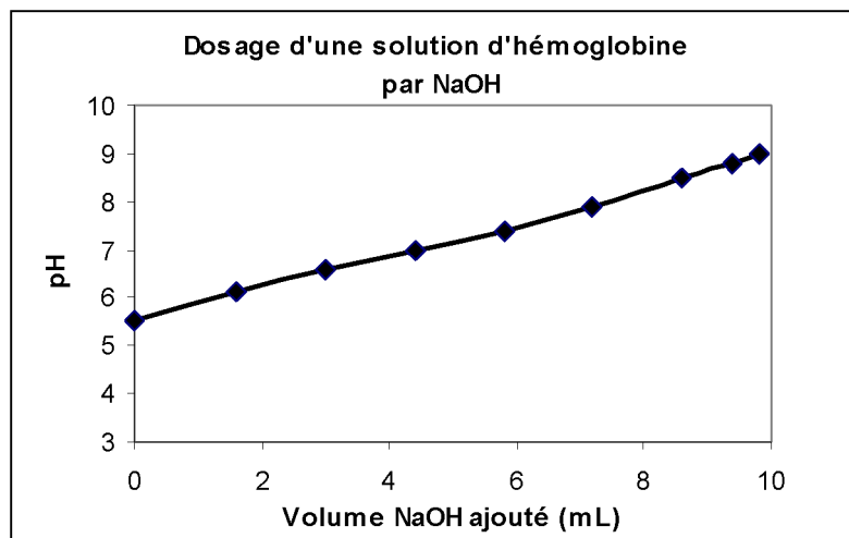
Graph 1 : Courbe de dosage basique d'une solution d'hémoglobine
