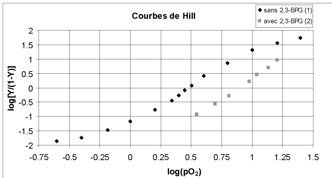
Graphe 5 : Courbes de Hill pour les solutions 1 et 2.
