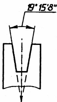
Умовне позначення кутового розміру.
