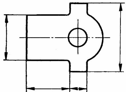
Взаємне розміщення виносних і розмірної ліній.
