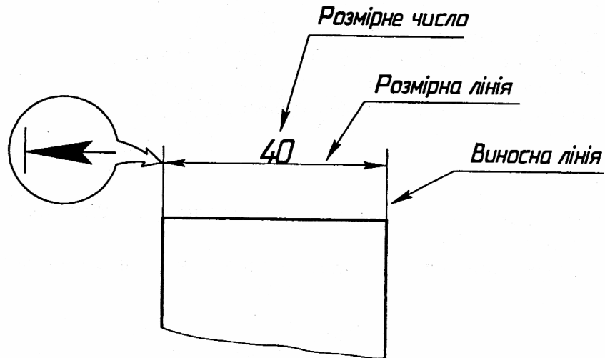
Елементи лінійного розміру на кресленні.
