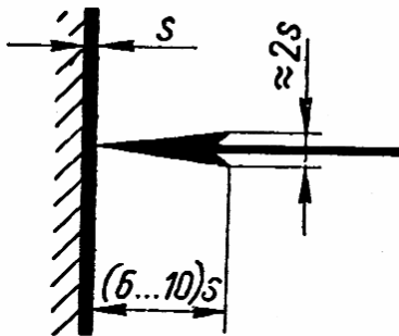
Розміри елементів стрілки.
