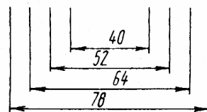
Розміщення розмірних чисел на паралельних розмірних лініях.
