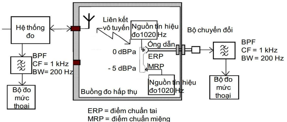
Hình 1 - Sơ đồ đo - Phương pháp giao thoa âm
