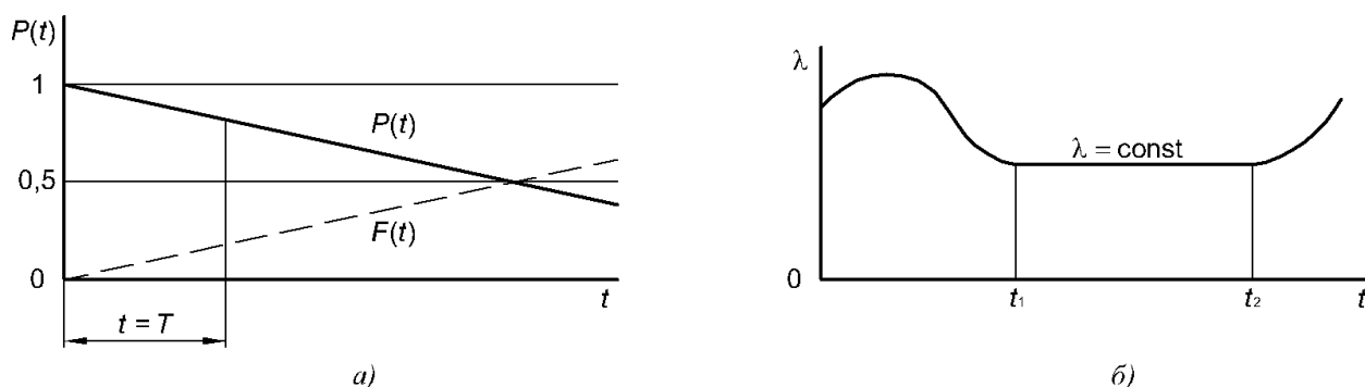
Рисунок 5.5 – Експоненціальний закон при раптових відмовах:
