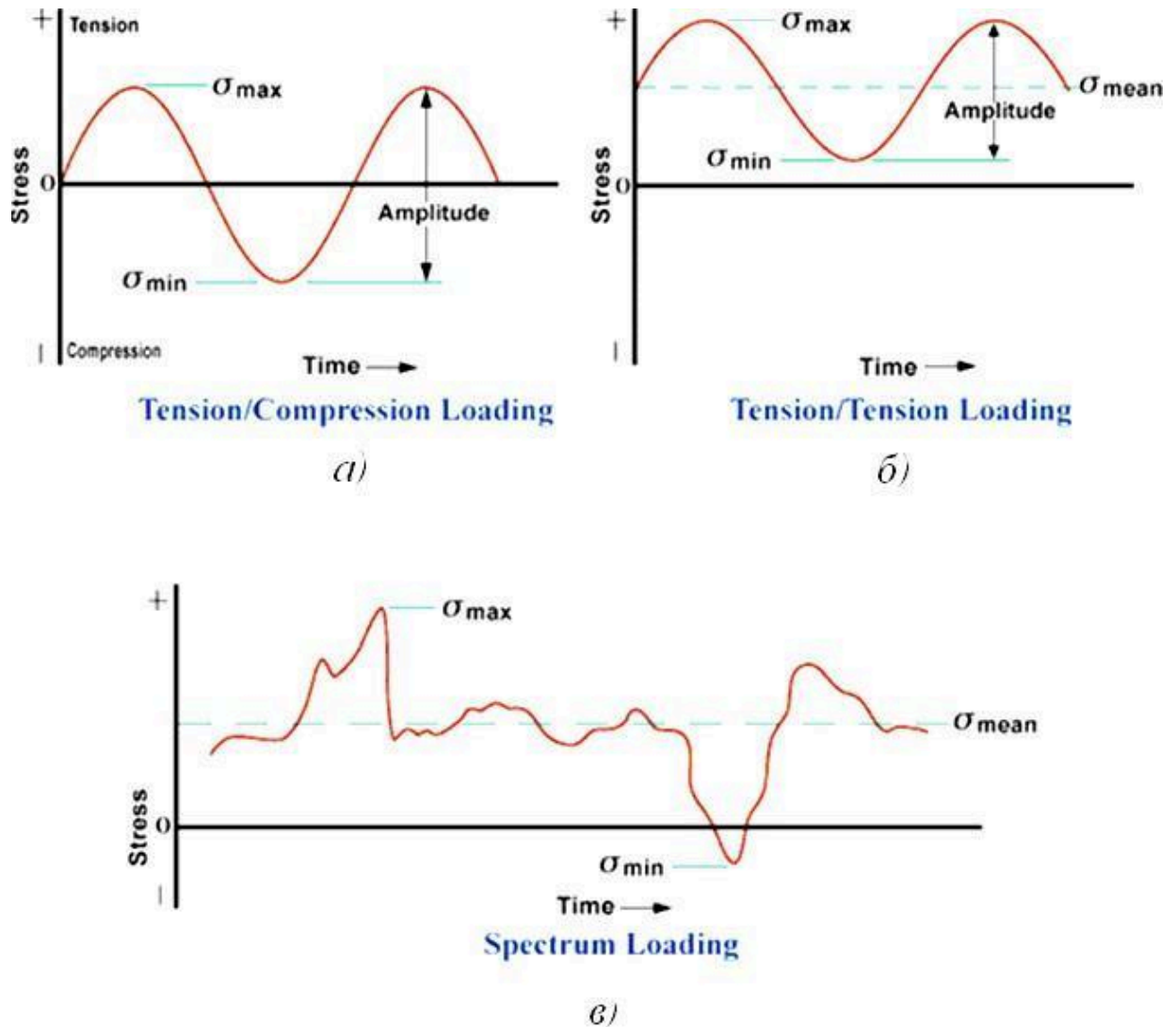
Рисунок 11.2 – Види циклічних навантажень за регулярністю: а і б – регулярні; в – нерегулярне
