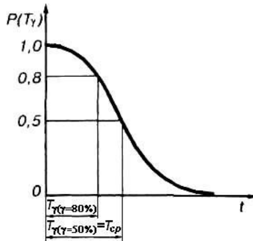
Рисунок 7.1 – Графоаналітичний метод визначення гамма-процентного напрацювання до відмови
