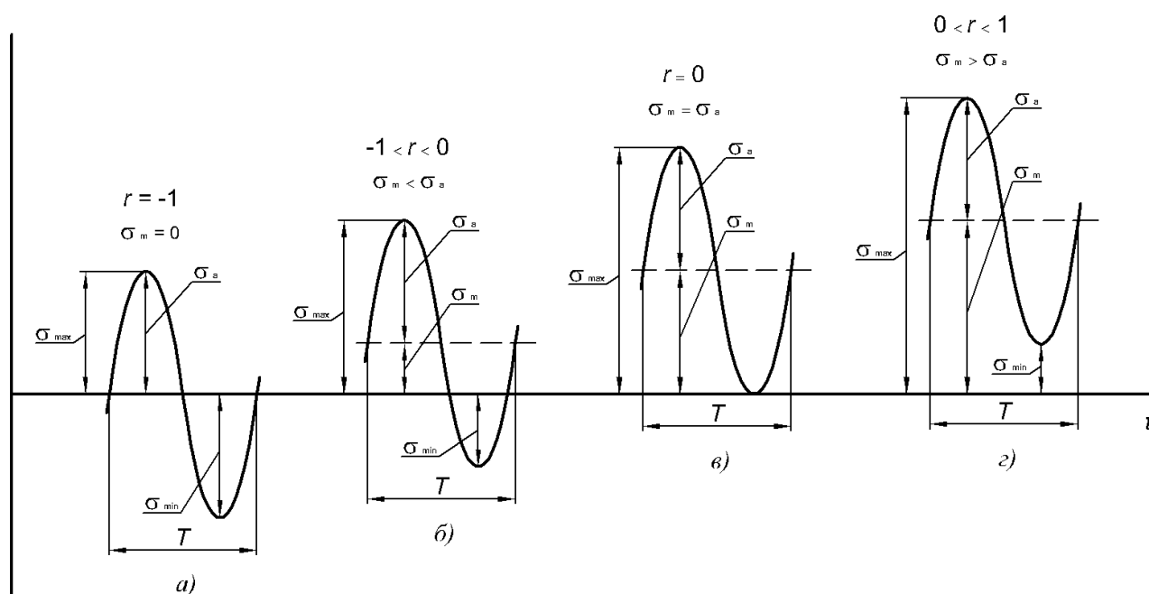
Рисунок 11.3 – Загальний вигляд синусоїдальних циклів:
