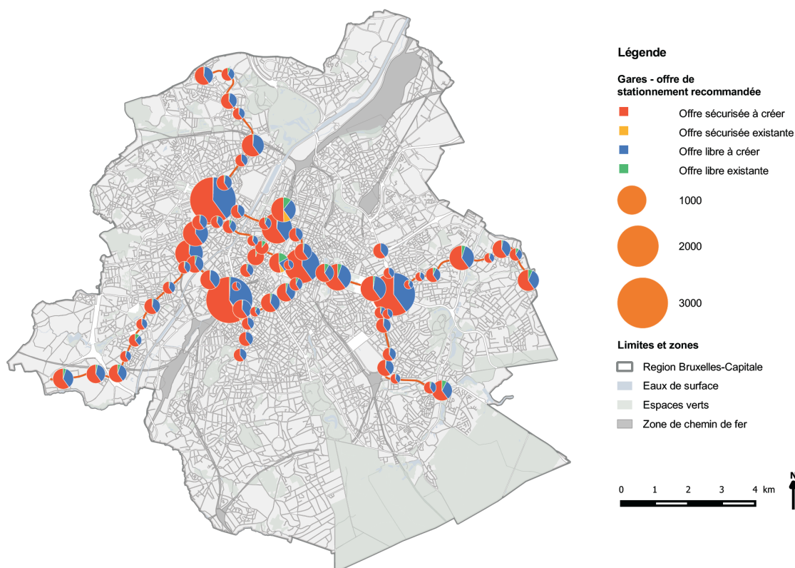
Figure 39 : Dimensionnement de l'offre de stationnement vélos dans les stations de métro et pré-métro
