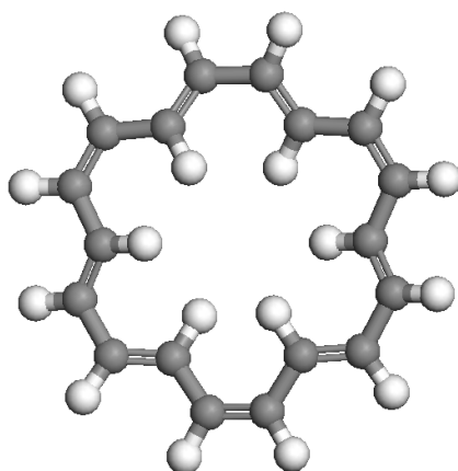
Figure 3 : Aromatique [18]-annulène
