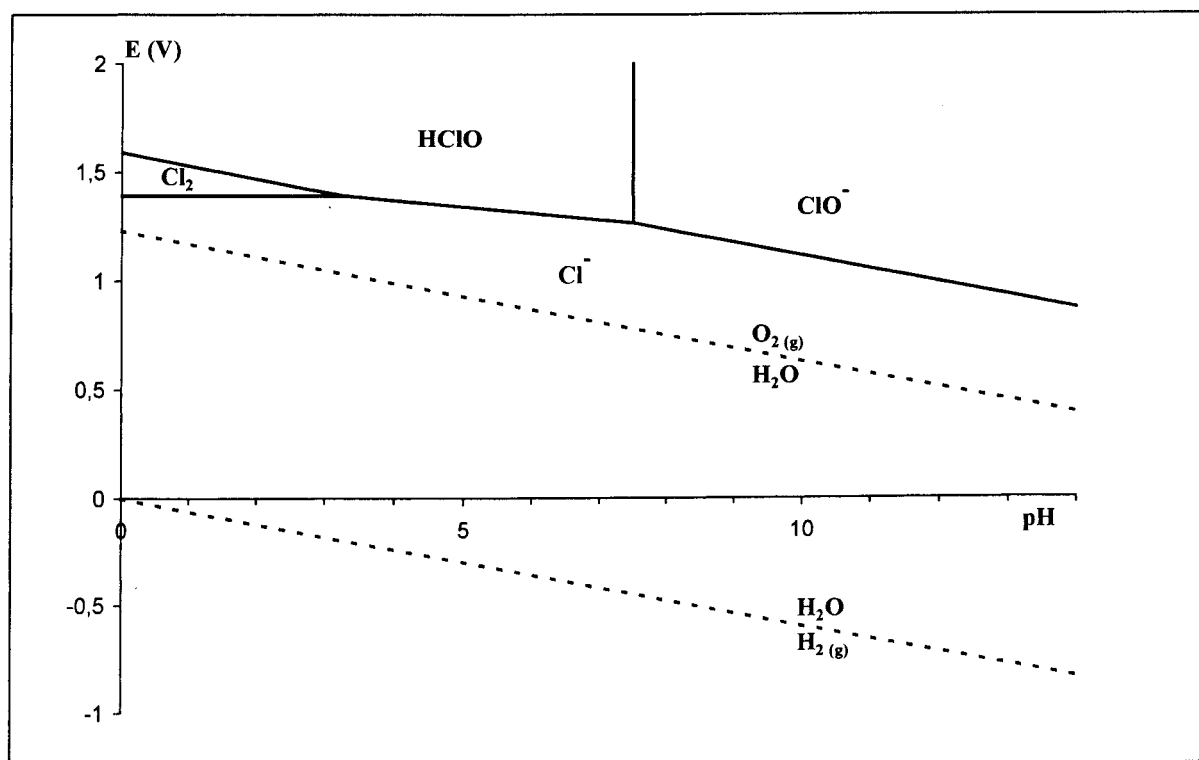
FIGURE 2 : Diagramme potentiel-pH du chlore (concentration de tracé 1 mol.L -1 ) et diagramme potentiel-pH de l'eau
