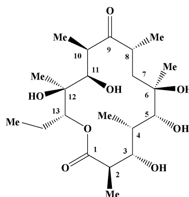
érythronolide B (1)
