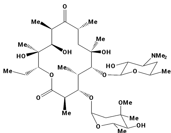
érythromycine A
