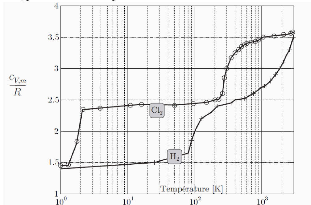
FIGURE 1 - Mesures de la capacité thermique molaire du dichlore ( \text{Cl}_2 ) et du dihydrogène ( \text{H}_2 ) gazeux en fonction de la température.
