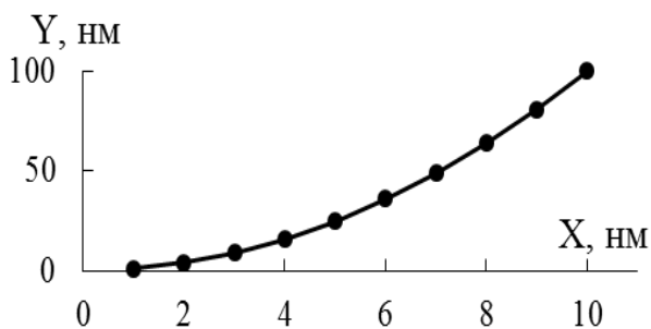
Рис. 1. Пример зависимости y=x^2 .
