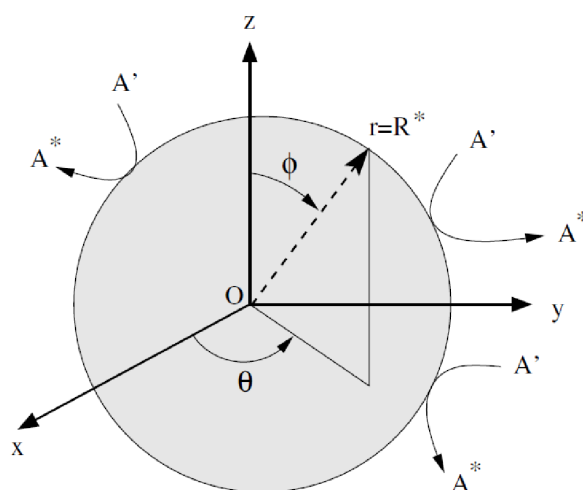
Figure 2 – Représentation géométrique de la distance d'approche du mécanisme de LINDEMANN-HINSHELWOOD : une molécule de A au centre du repère ( O, \hat{u}_r, \hat{u}_\theta, \hat{u}_\phi ) ne peut être approchée à moins de r = R^* par une autre molécule. Se reporter au texte pour les notations.
