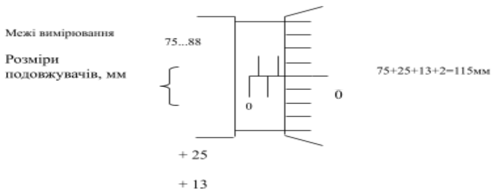
Рис 2. Зразок відліку на шкалах мікрометричного нутроміра для розміру 115 мм
