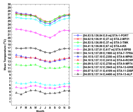
Gambar 1. Temperatur rata-rata bulanan AWS PTFI per ketinggian. (10pt)
