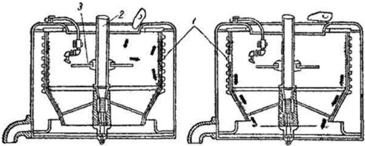
Рис. 5.3. Саморозвантажна центрифуга:
