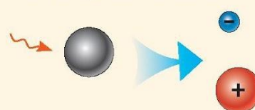
Рис. 7.2. Деякі види йонізації газів
