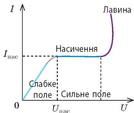
Рис. 7.4. Вольт-амперна характеристика (ВАХ) газового розряду
