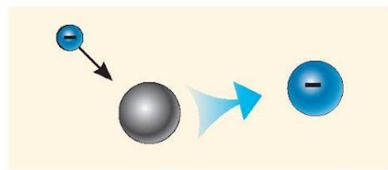
Рис. 7.1. Схема утворення негативних йонів у газах
