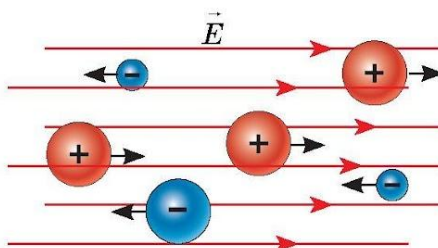
Рис. 7.3. В йонізованому газі за наявності електричного поля виникає напрямлений рух вільних заряджених частинок — електричний струм
